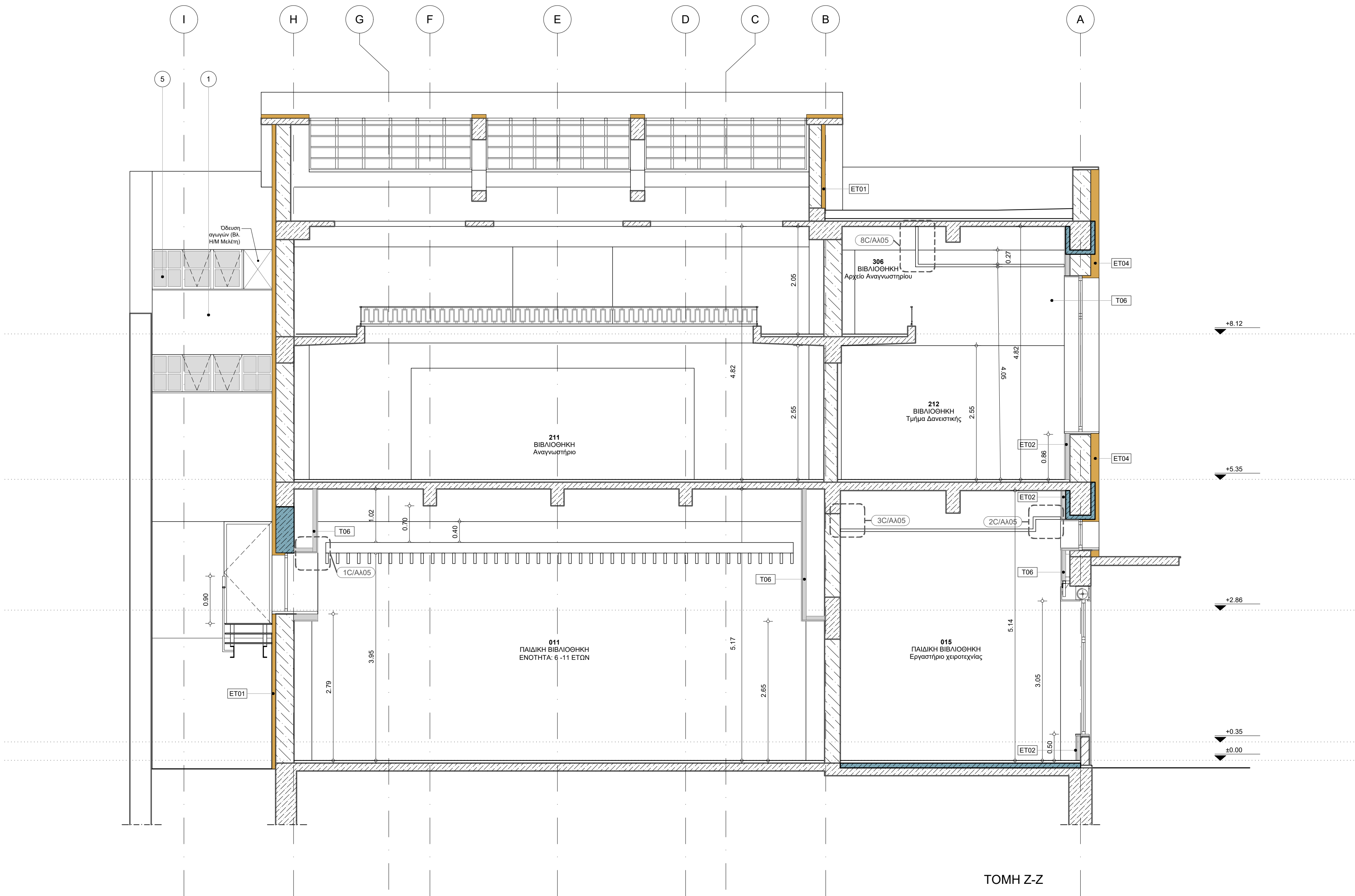
ΤΟΜΗ Z-Z
