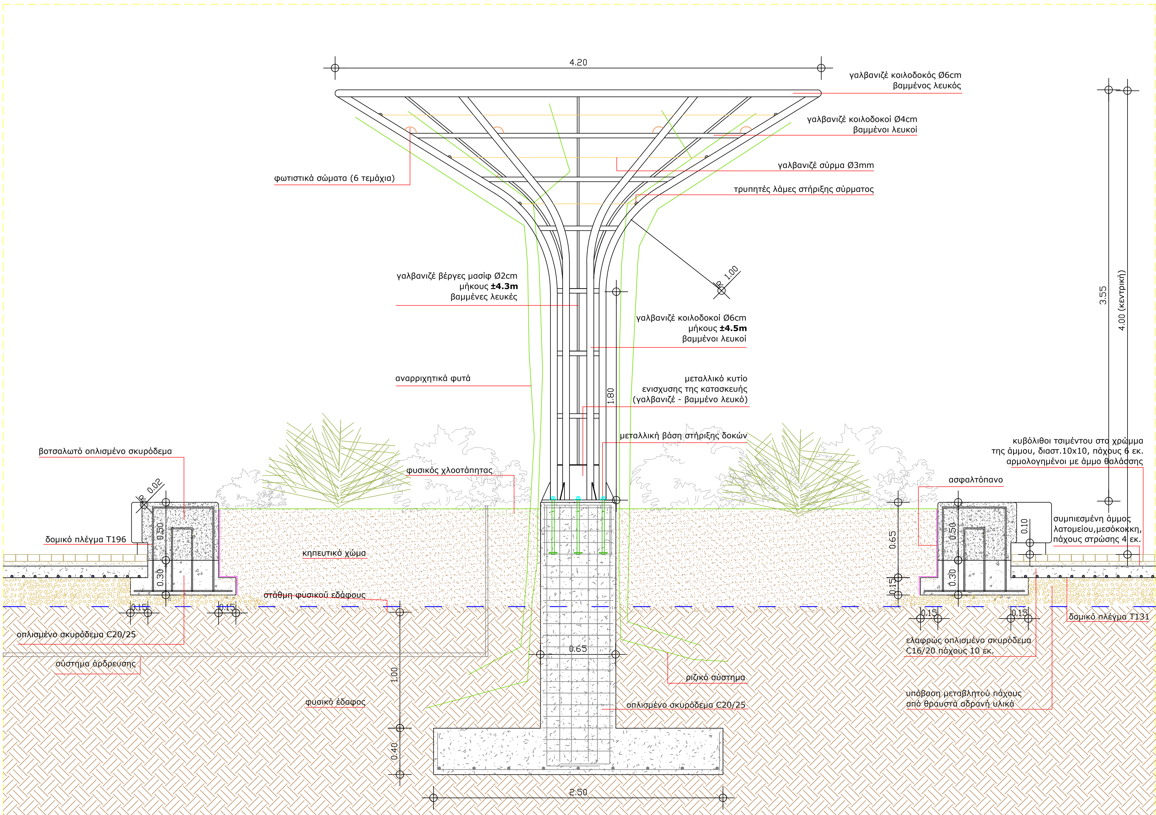
ΤΟΜΗ ΚΕΝΤΡΙΚΗΣ ΠΕΡΓΚΟΛΑΣ - ΠΕΡΙΜΕΤΡΙΚΟΥ ΚΑΘΙΣΤΙΚΟΥ
