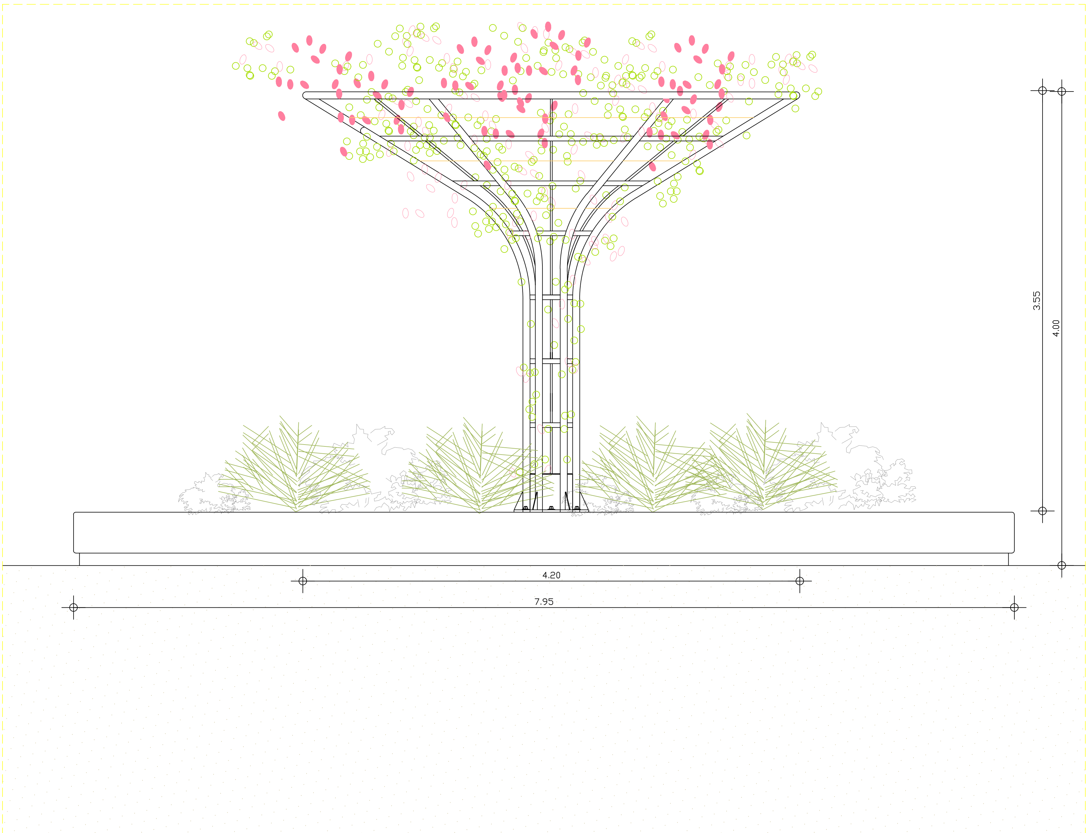
ΩΨΗ ΚΕΝΤΡΙΚΗΣ ΠΕΡΓΚΟΛΑΣ - ΠΕΡΙΜΕΤΡΙΚΟΥ ΚΑΘΙΣΤΙΚΟΥ
