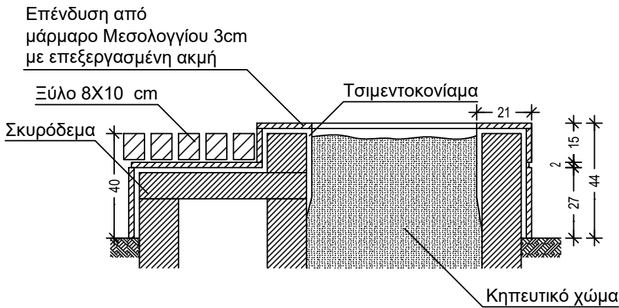
ΤΟΜΗ
