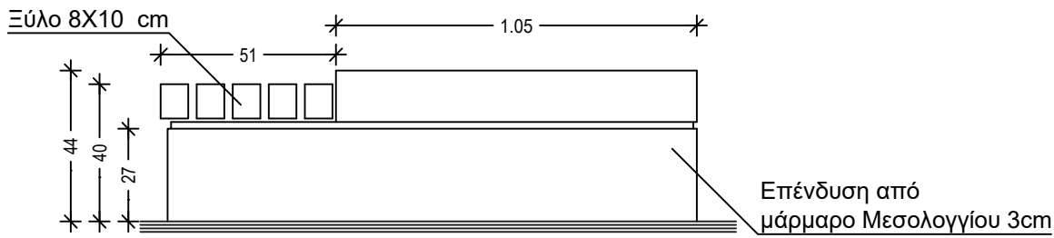
ΟΨΗ
