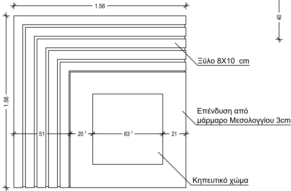
ΚΑΤΟΨΗ
