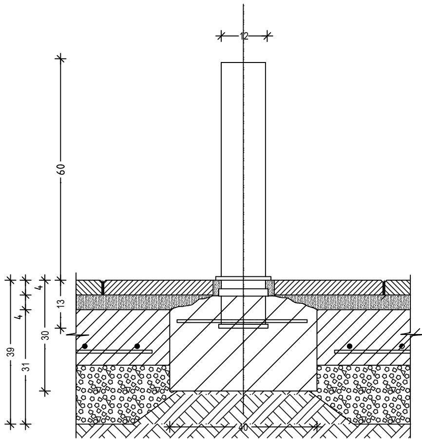
ΣΤΑΘΕΡΗ ΑΝΟΞΕΙΔΩΤΗ ΜΠΑΡΑ (ΔΙΑΒΑΣΗ ΠΕΖΩΝ) ΛΕΠΤΟΜΕΡΕΙΑ Λ1 ΚΛΙΜΑΚΑ 1/10
