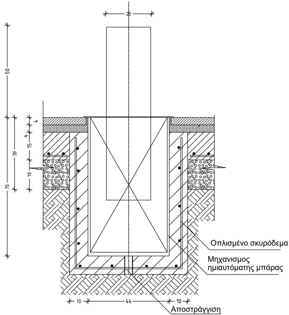
ΒΥΘΙΖΟΜΕΝΗ ΗΜΙΑΥΤΟΜΑΤΗ ΑΝΟΞΕΙΔΩΤΗ ΜΠΑΡΑ (ΕΛΕΓΧΟΜΕΝΗ ΔΙΑΒΑΣΗ ΑΥΤΟΚΙΝΗΤΩΝ) ΛΕΠΤΟΜΕΡΕΙΑ Λ4 ΚΛΙΜΑΚΑ 1/10
