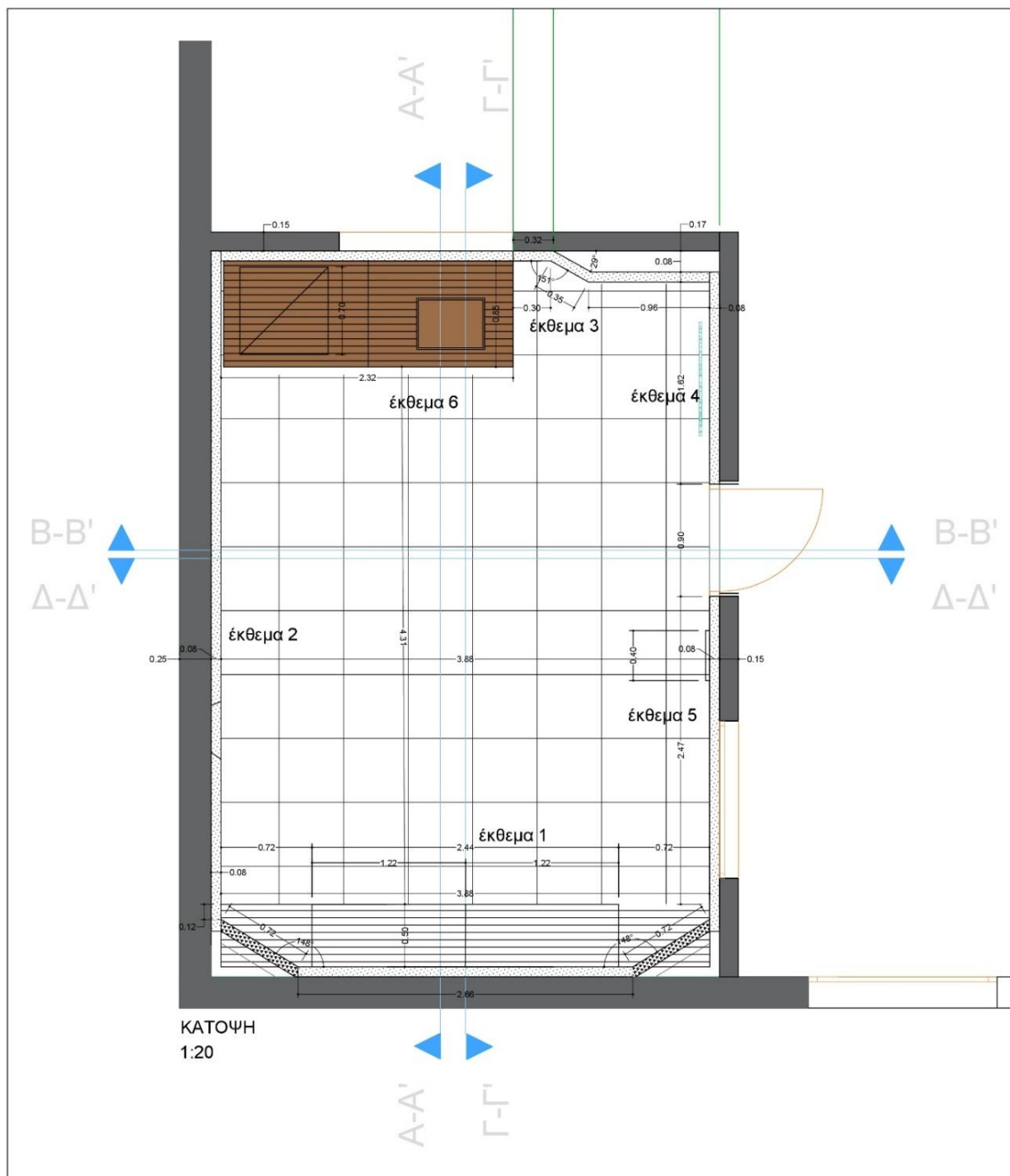
Κάτοψη εκθεσιακού χώρου Κέντρου Πληροφόρησης Παναχαϊκού Όρους
