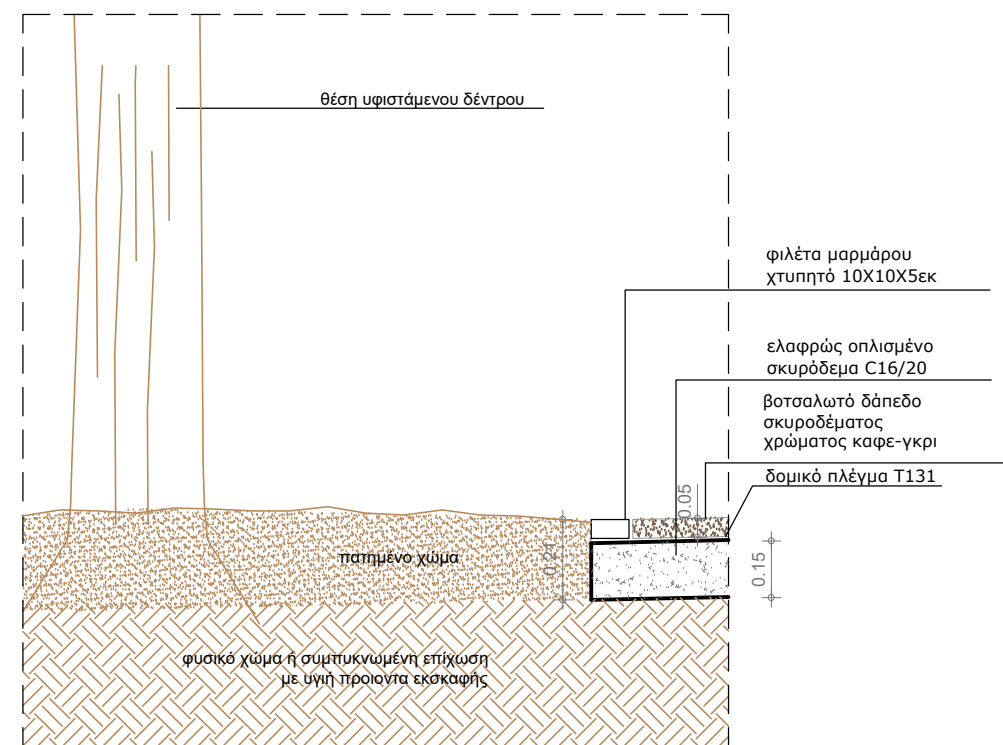
ΤΟΜΗ
