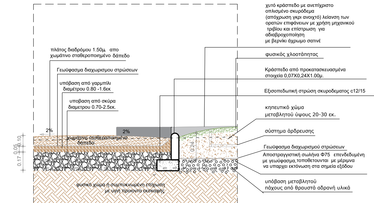
ΤΟΜΗ
