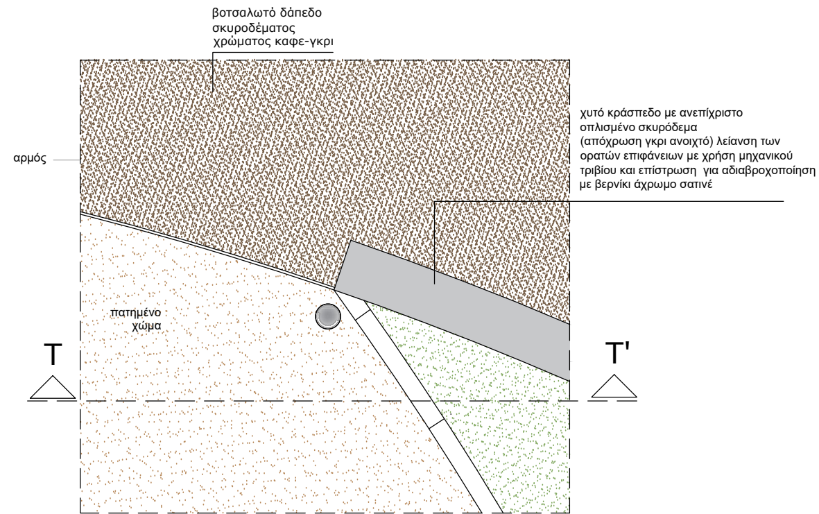
ΚΑΤΟΨΗ
