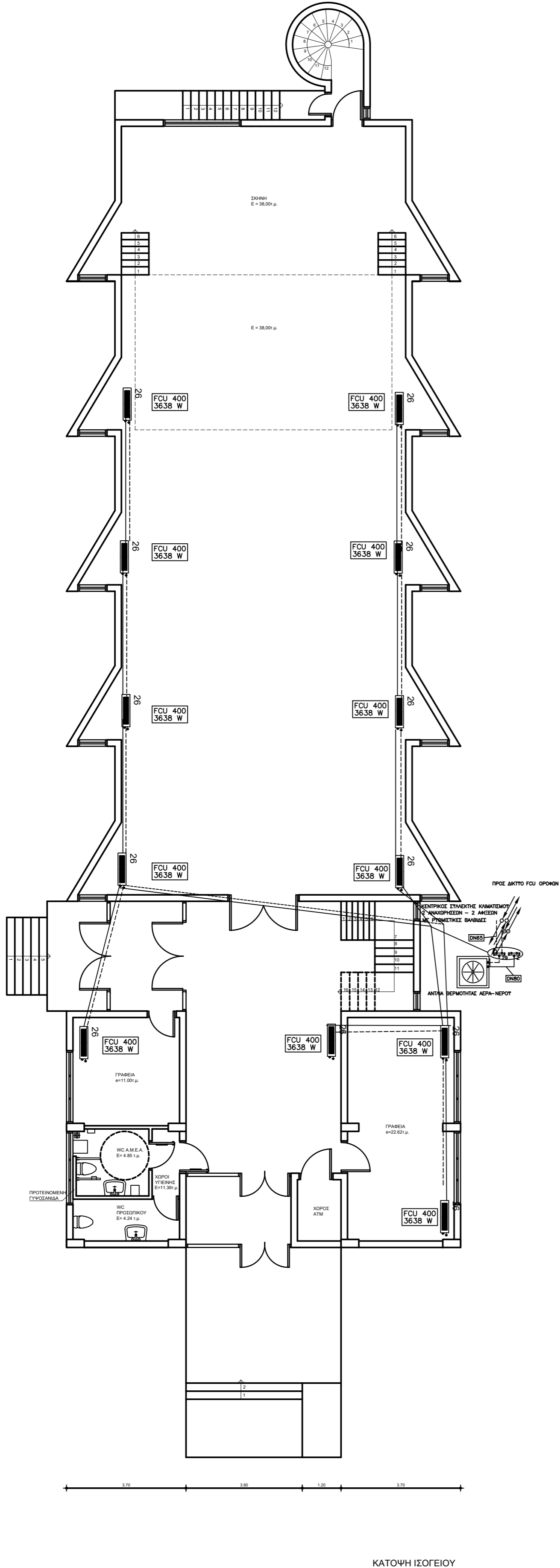
ΚΑΤΟΨΗ ΙΣΟΓΕΙΟΥ
