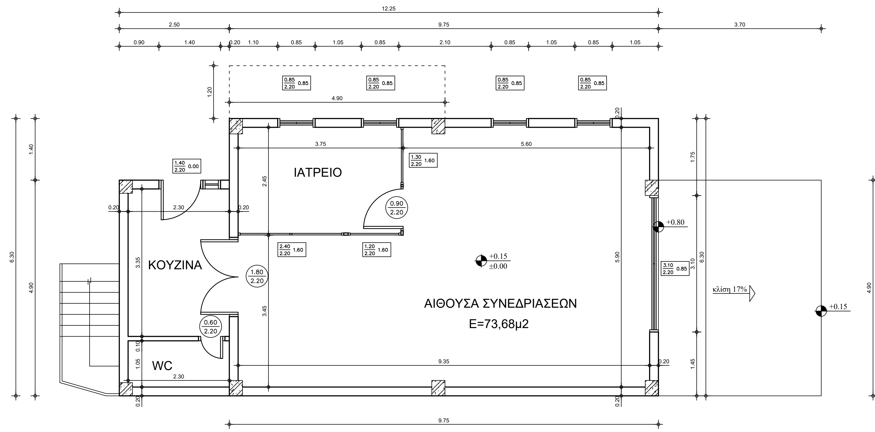
ΚΑΤΟΨΗ ΙΣΟΓΕΙΟΥ
