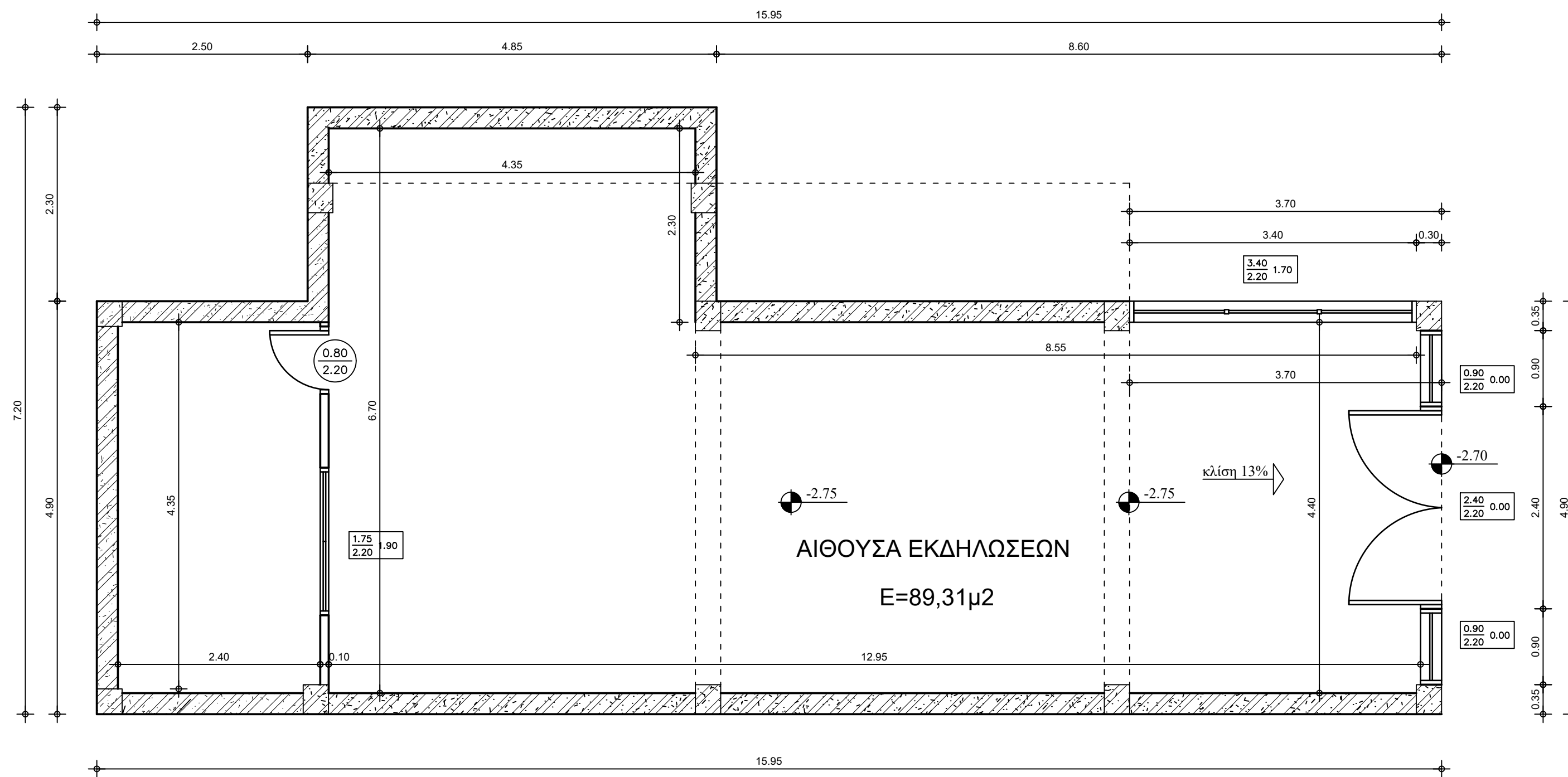
ΚΑΤΟΨΗ ΥΠΟΓΕΙΟΥ
