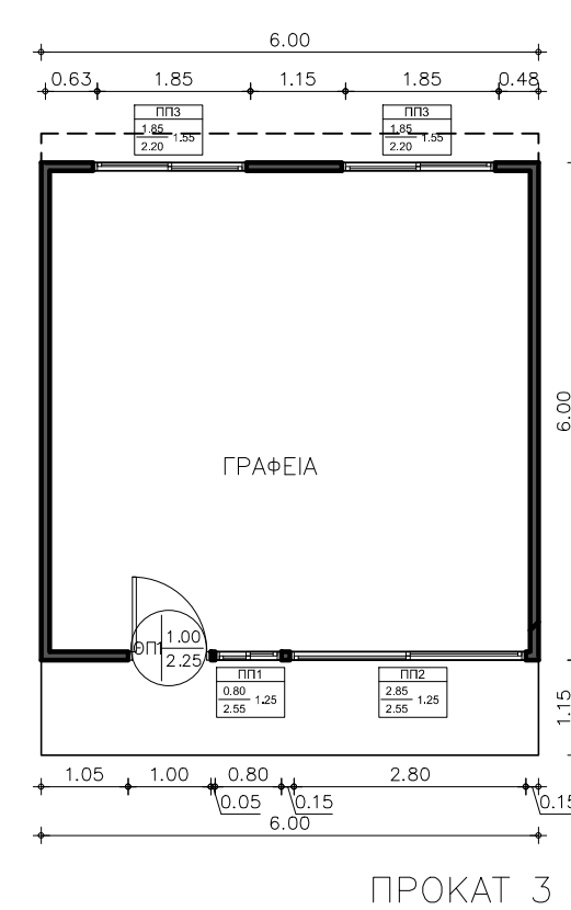
ΚΑΤΟΨΕΙΣ ΙΣΟΓΕΙΟΥ
