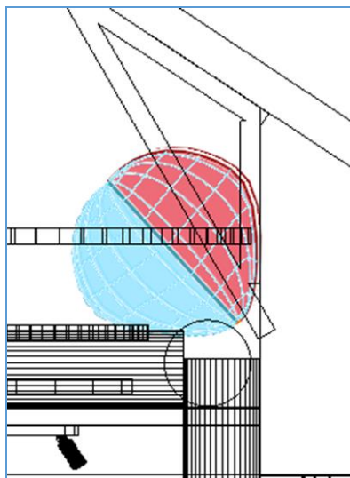
Εικόνα 4: Θέση ταινίας LED σε σχέση με τον τοίχο και τον αεραγωγό
