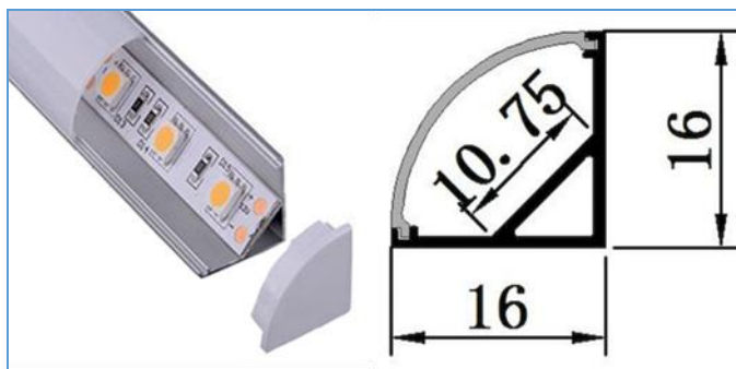
Εικόνα 3: Ενδεικτικό προφίλ αλουμινίου με διαστάσεις
