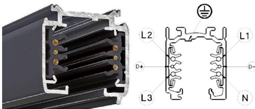
Εικόνα 2: Ράγα Dali σε τομή.
