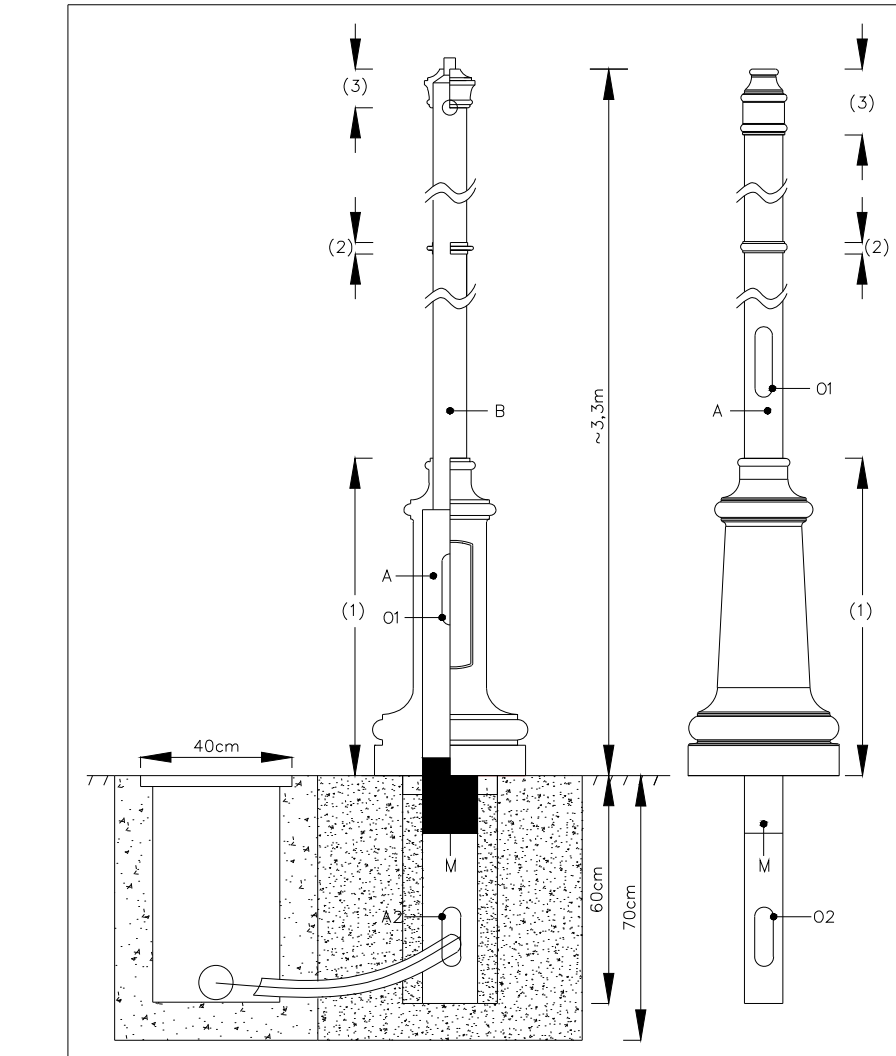
ΛΕΠΤΟΜΕΡΕΙΑ ΕΔΡΑΣΗΣ ΕΠΙΣΤΥΛΟΥ ΦΩΤΙΣΤΙΚΟΥ ΚΛΙΜΑΚΑ 1:20
