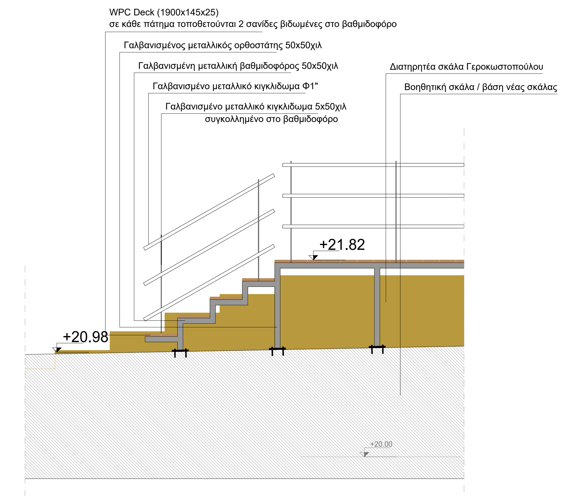
ΛΕΠΤΟΜΕΡΕΙΑ ΞΥΛΙΝΟΥ ΤΜΗΜΑΤΟΣ ΝΕΑΣ ΣΚΑΛΑΣ ΚΛΙΜΑΚΑ 1:20
